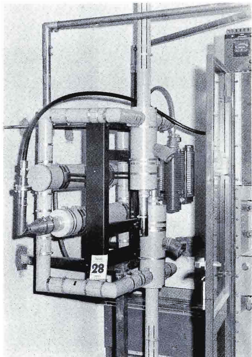
FIG. 9 11KW Notch Diplexer adjoins TTL-500AH TV Transmitter.
